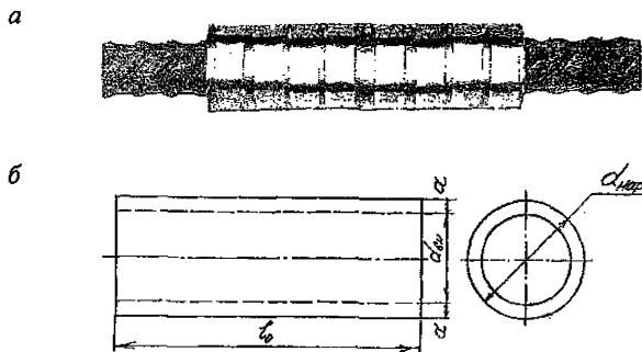
Рисунок В.1: a – опрессованный стык построечного изготовления, произведенный на мобильном оборудовании многократным поперечным деформированием соединительной муфты с промежутками, b – соединительная муфта для опрессованных стыков
